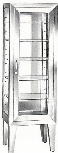
〔仕様〕 材質：ステンレス製 SUS-304 棚板：5枚 G/ガラス S/ステンレス
